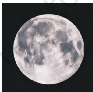
Moon
